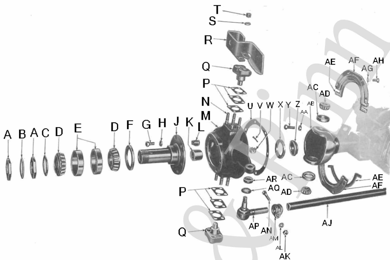
Steuergehäuse / Steering knuckle
