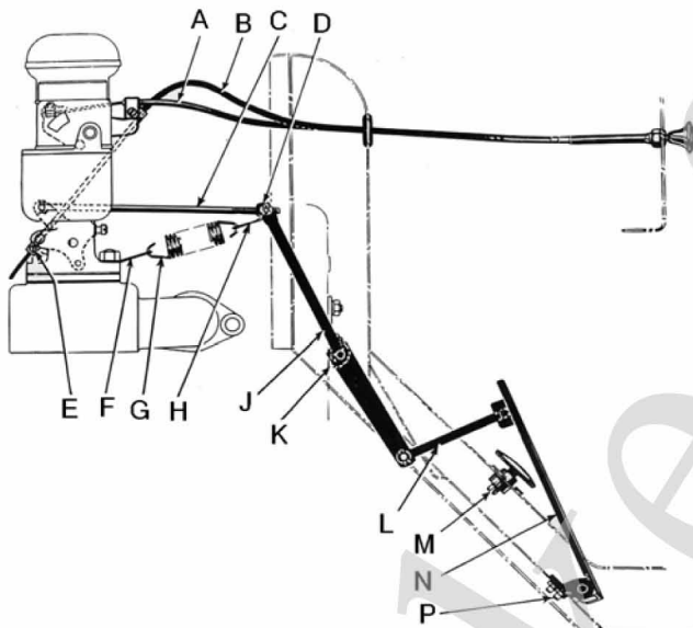
Gasgestänge / Throttle & choke control
