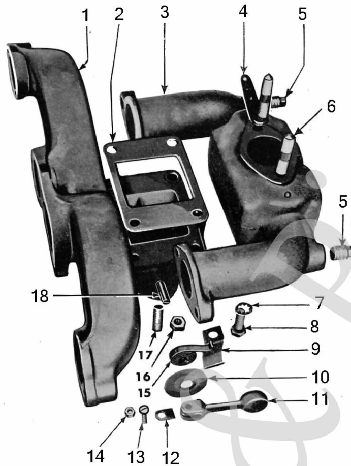
Auspuffkrümmer / Exhaust manifold
