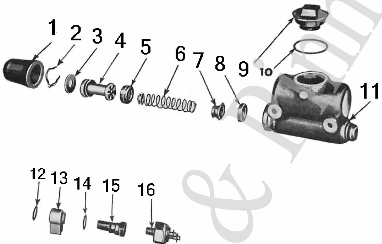
Hauptbremszylinder / Brake master cylinder
