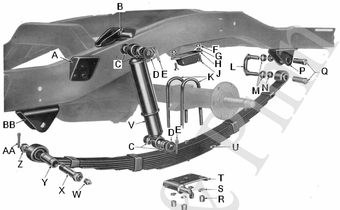
Blattfeder hinten / Rear spring
