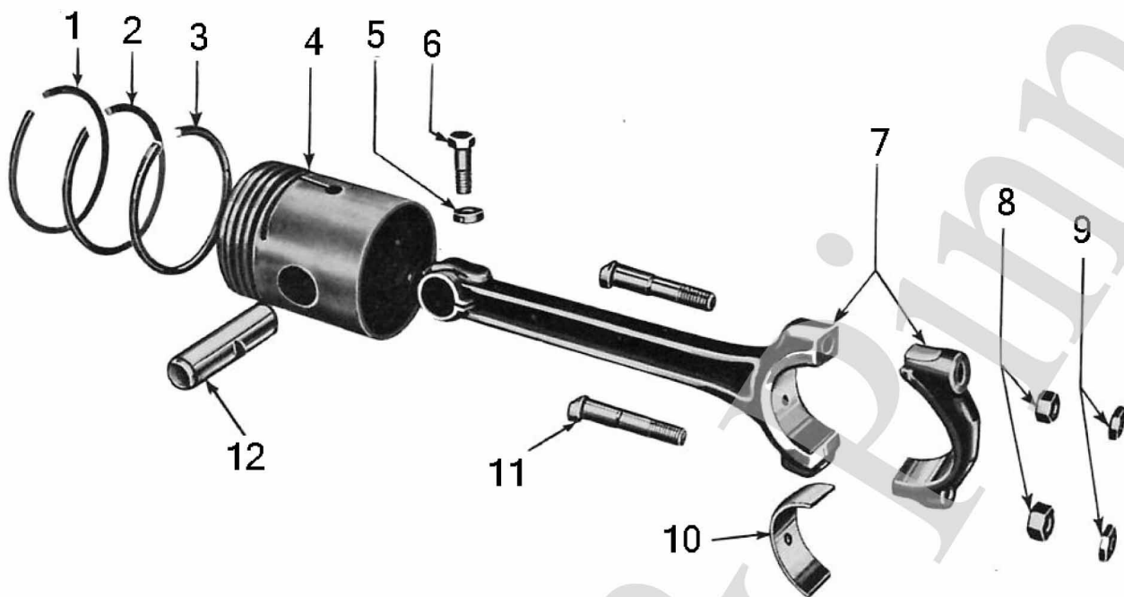
Kolben & Pleuel / Piston & Rod
