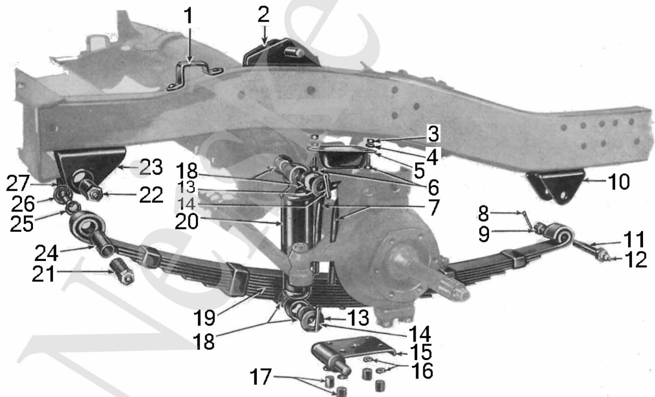
Blattfeder vorn / Front spring
