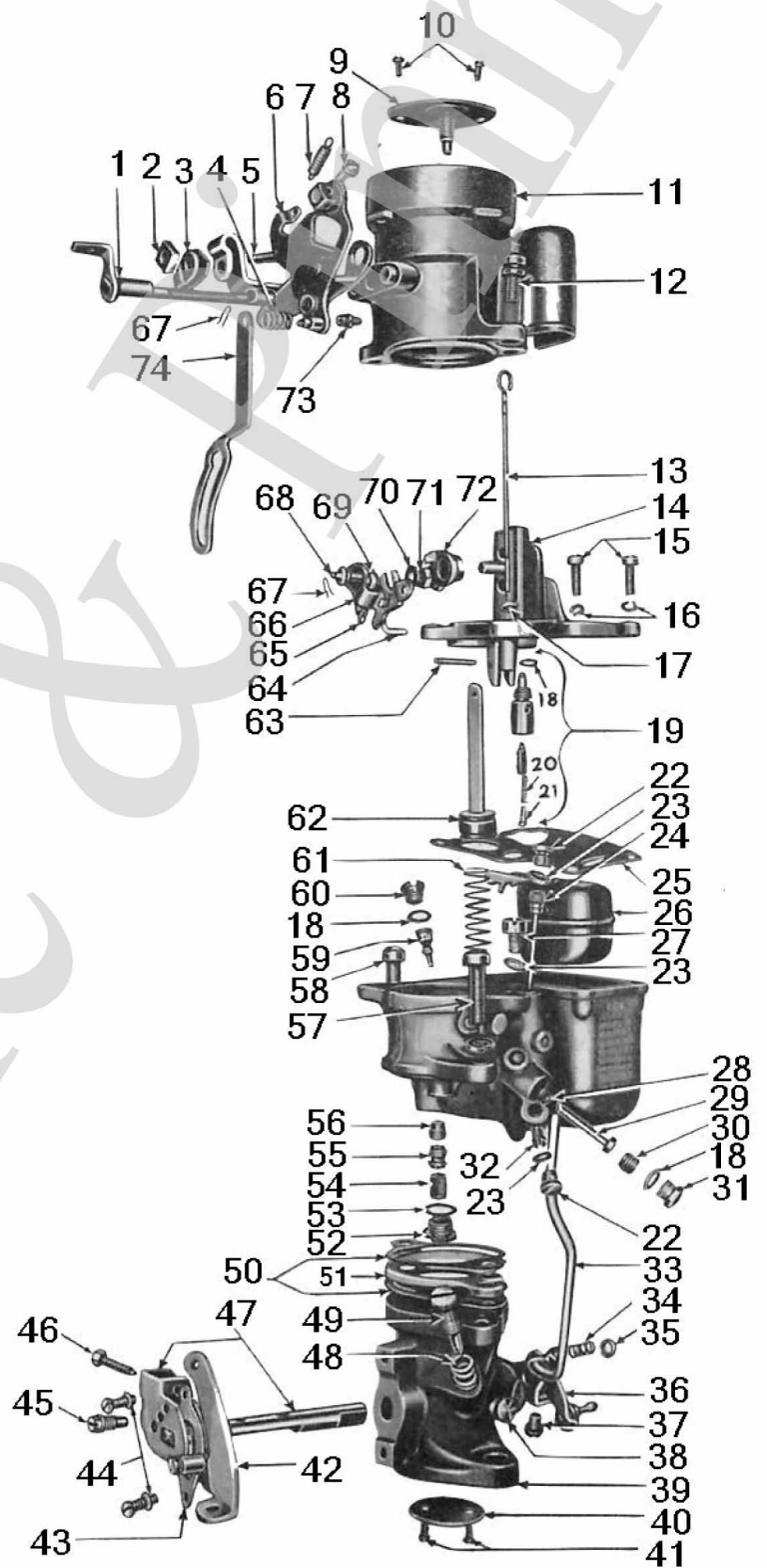
Gasgestänge / Throttle & choke control
