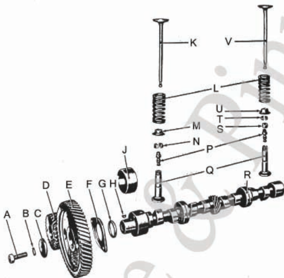
Nockenwelle / Camshaft
