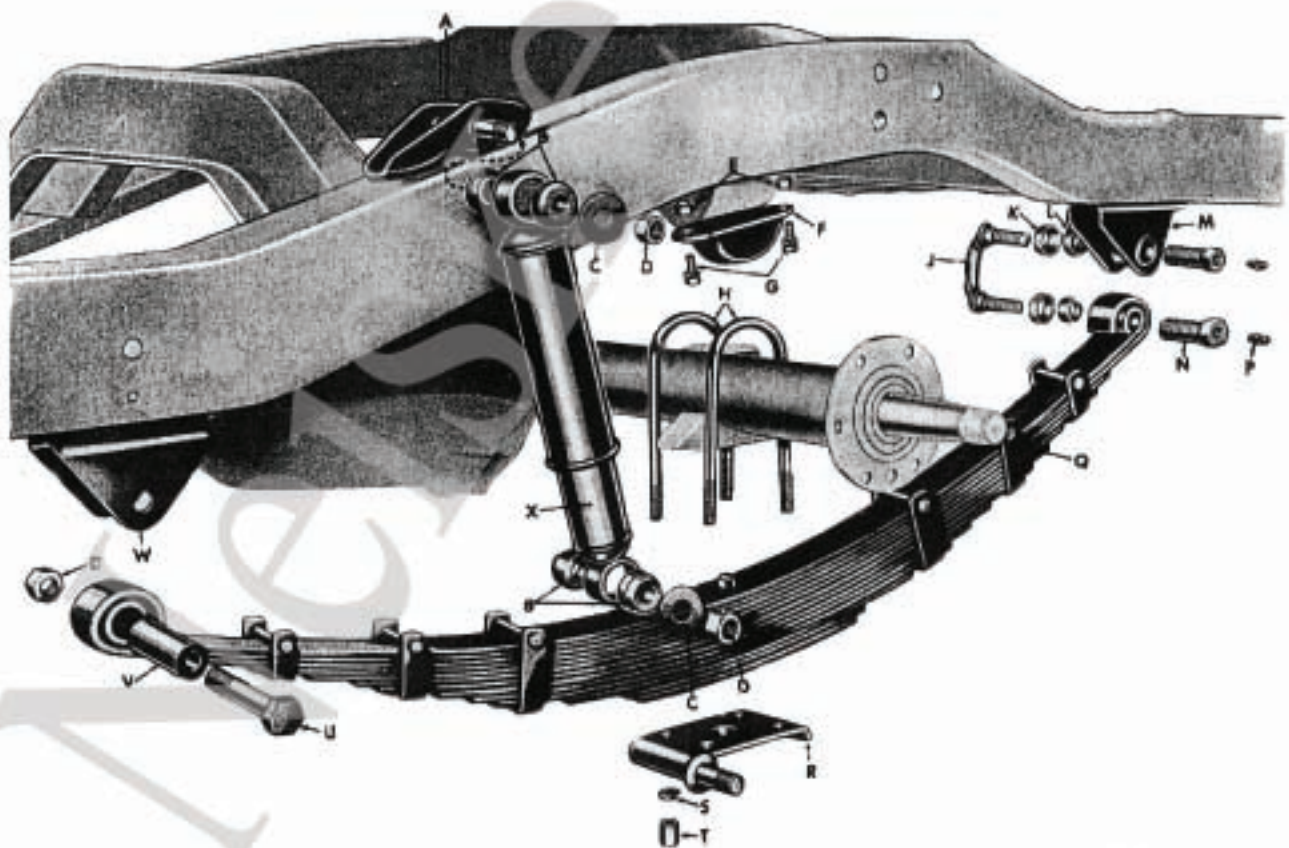
Blattfeder hinten / Rear spring
