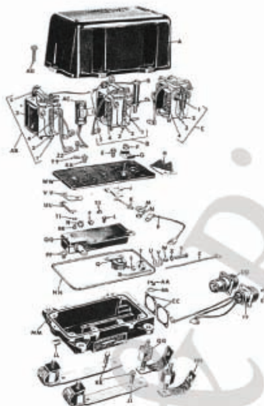
Regler / Regulator 24V
