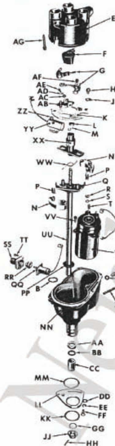
Zündverteiler / Distributor
