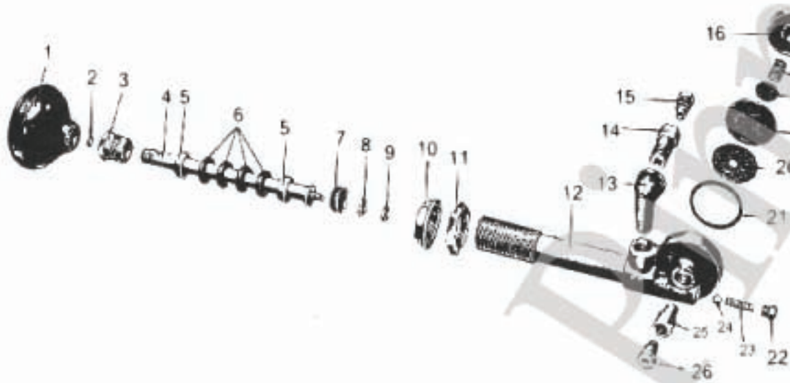
Handbenzinpumpe / Primer pump
