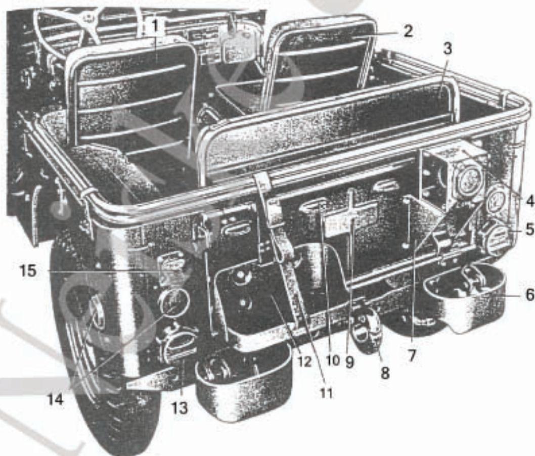
Karosserie hinten / Body rear
