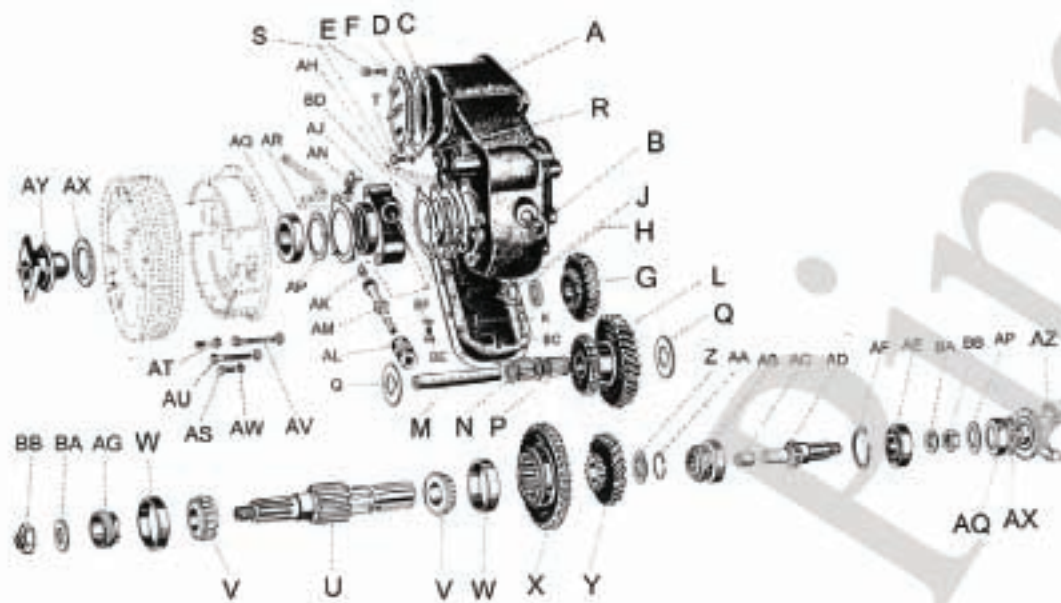
Untersetzungsgetriebe / Transfer case
