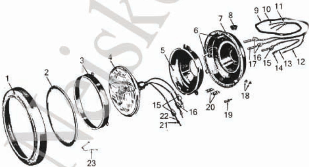
Scheinwerfer / Head light
