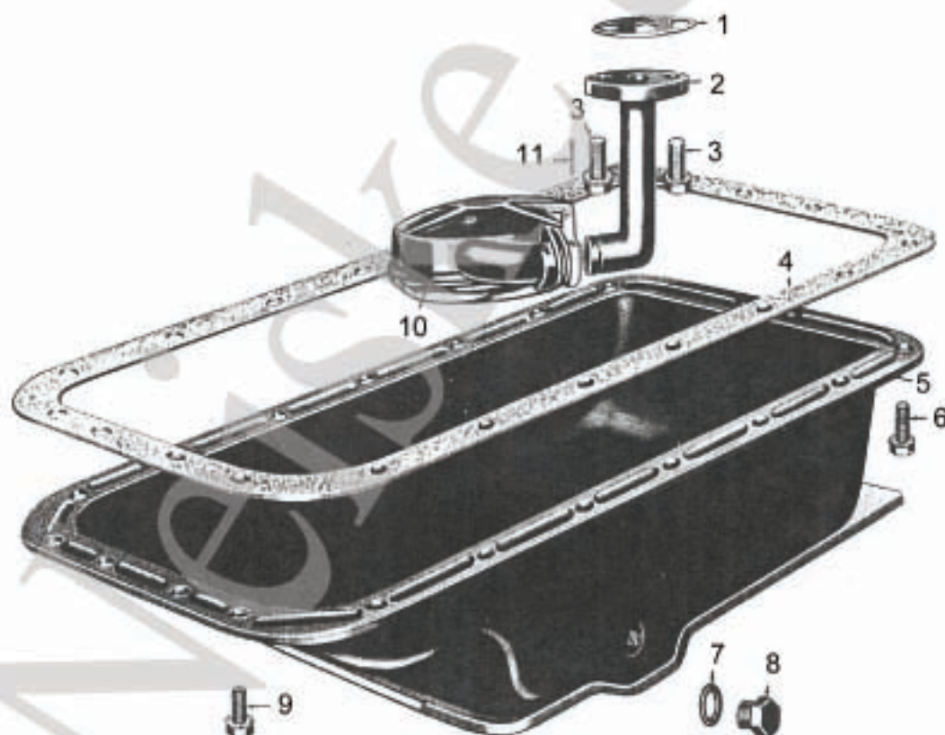
Ölwanne / Oil pan
