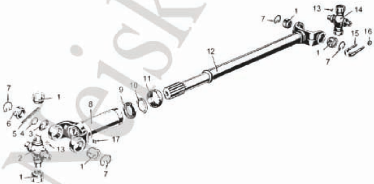
Kardanwelle hinten / Propeller shaft rear
