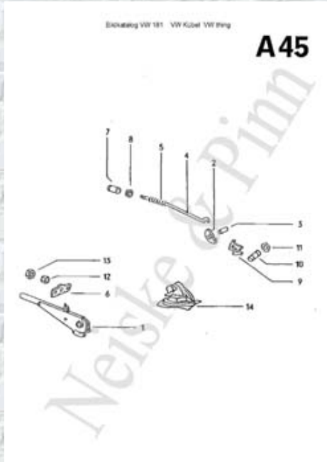
Page 45A Handbremshebel
