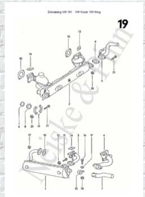
Page 19 Abgasanlage
