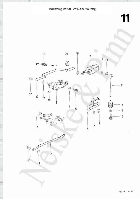
Page 11 Kühlluftregulierung
