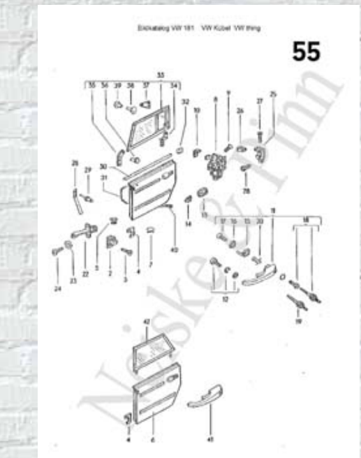
Page 55 Türen + Steckfenster
