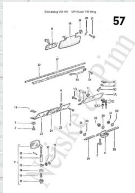
Page 57 Schalttafel Rückspiegel
