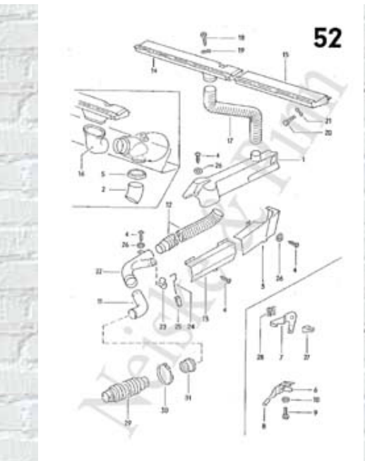
Page 52 Verteilung Warmluft
