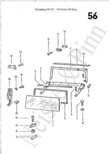
Page 56 Fensterrahmen Fensterscheiben
