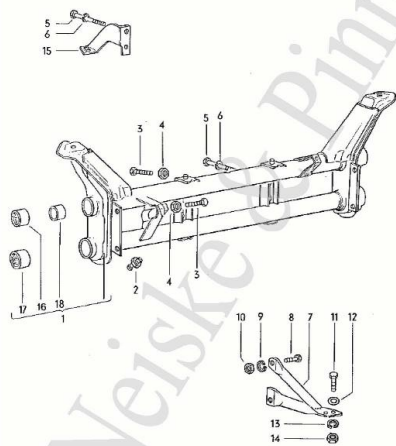
Page 26 Vorderachse
