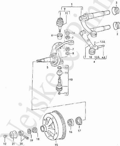
Page 26-1 Tragarm Achsschenkel
