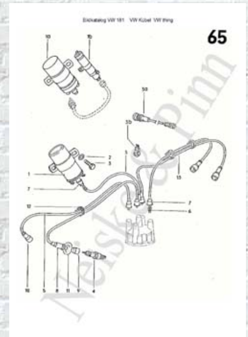
Page 65 Zündkabel
