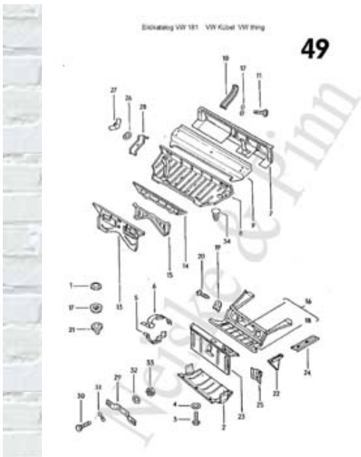
Page 49 Bleche Vorderteil
