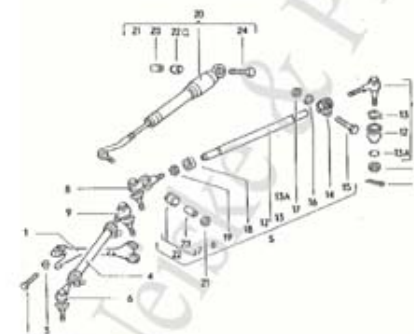
Page 29 Spurstange Lenkungsdämpfer
