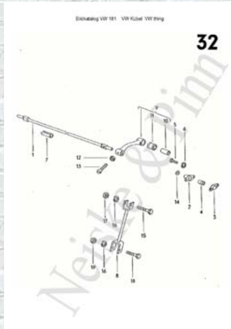
Page 32 Stabilisator hinten
