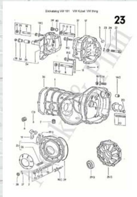
Page 23 Getriebe
