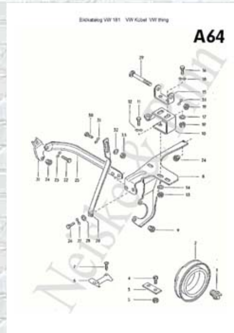
Page 64A Befestigung Lichtmaschine
