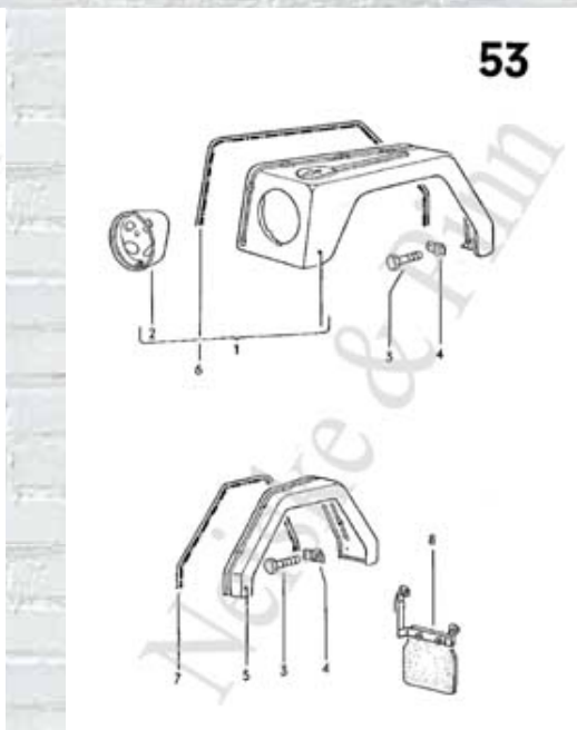
Page 53 Kotflügel
