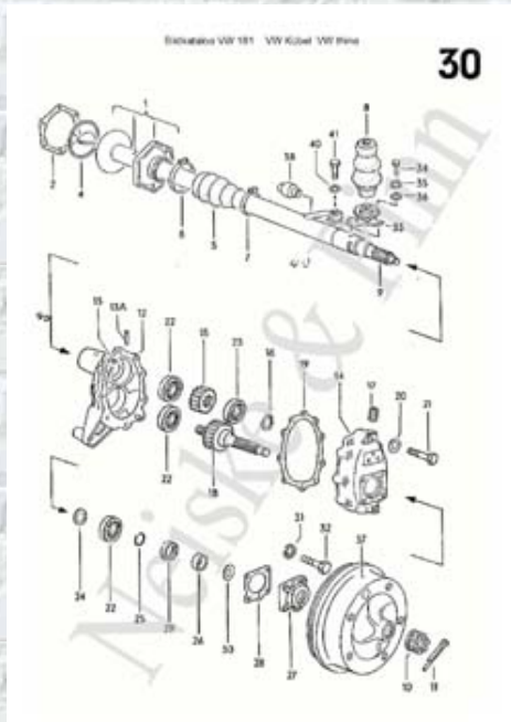
Page 30 Achse hinten Pendelachse
