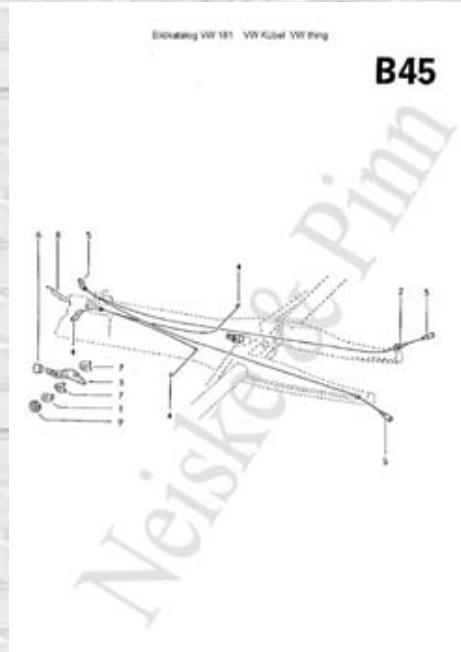
Page 45B Heizungszüge
