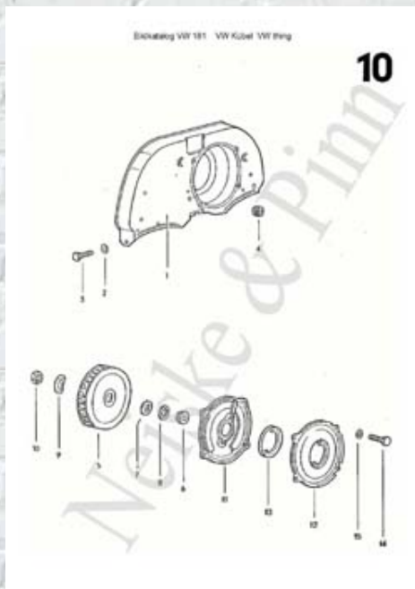
Page 10 Kühlgebläsegehäuse
