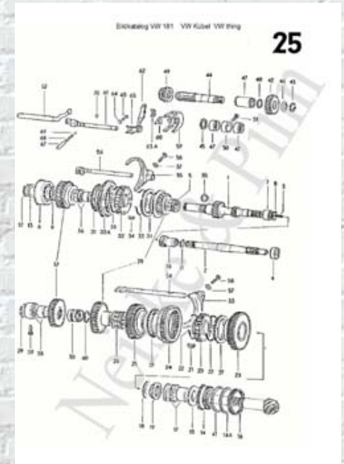
Page 25 Getriebe Zahnräder Wellen
