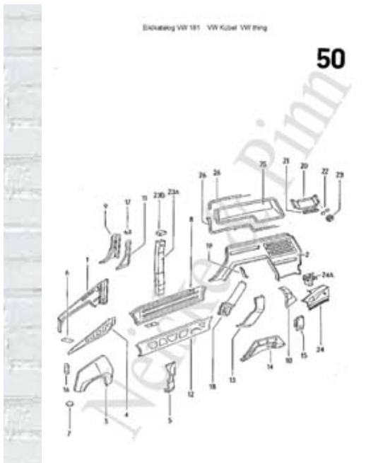
Page 50 Seitenteil Schweller
