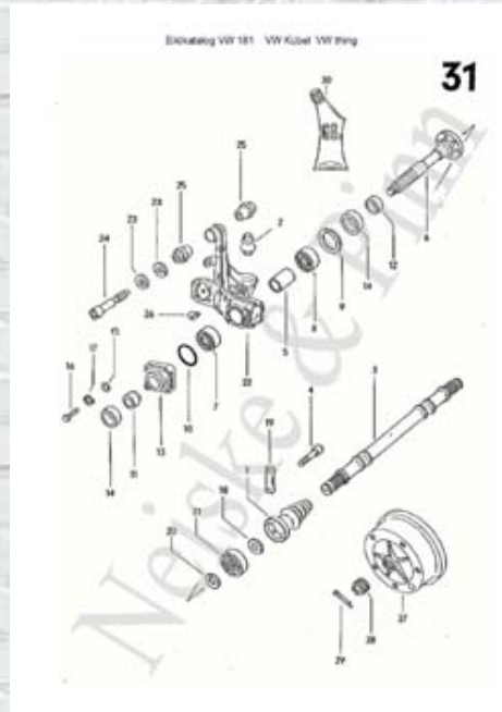
Page 31 Achse hinten Schräglenker
