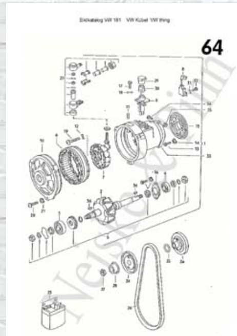
Page 64 Drehstrom-Lichtmaschine
