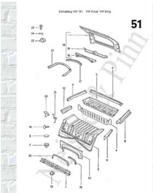
Page 51 Abschlussbleche hinten
