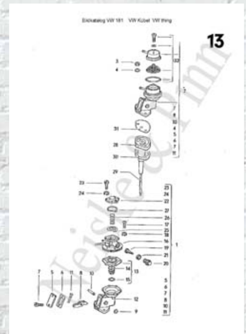
Page 13 Kraftstoffpumpe
