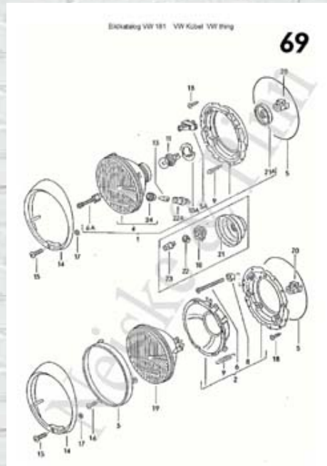
Page 69 Scheinwerfer ab 73
