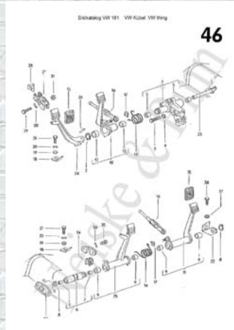
Page 46 Pedale Bremse + Kupplung
