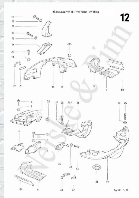
Page 12 Abdeckblech
