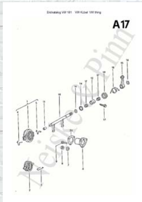
Page 17A Ausrücklager, Ausrückwelle
